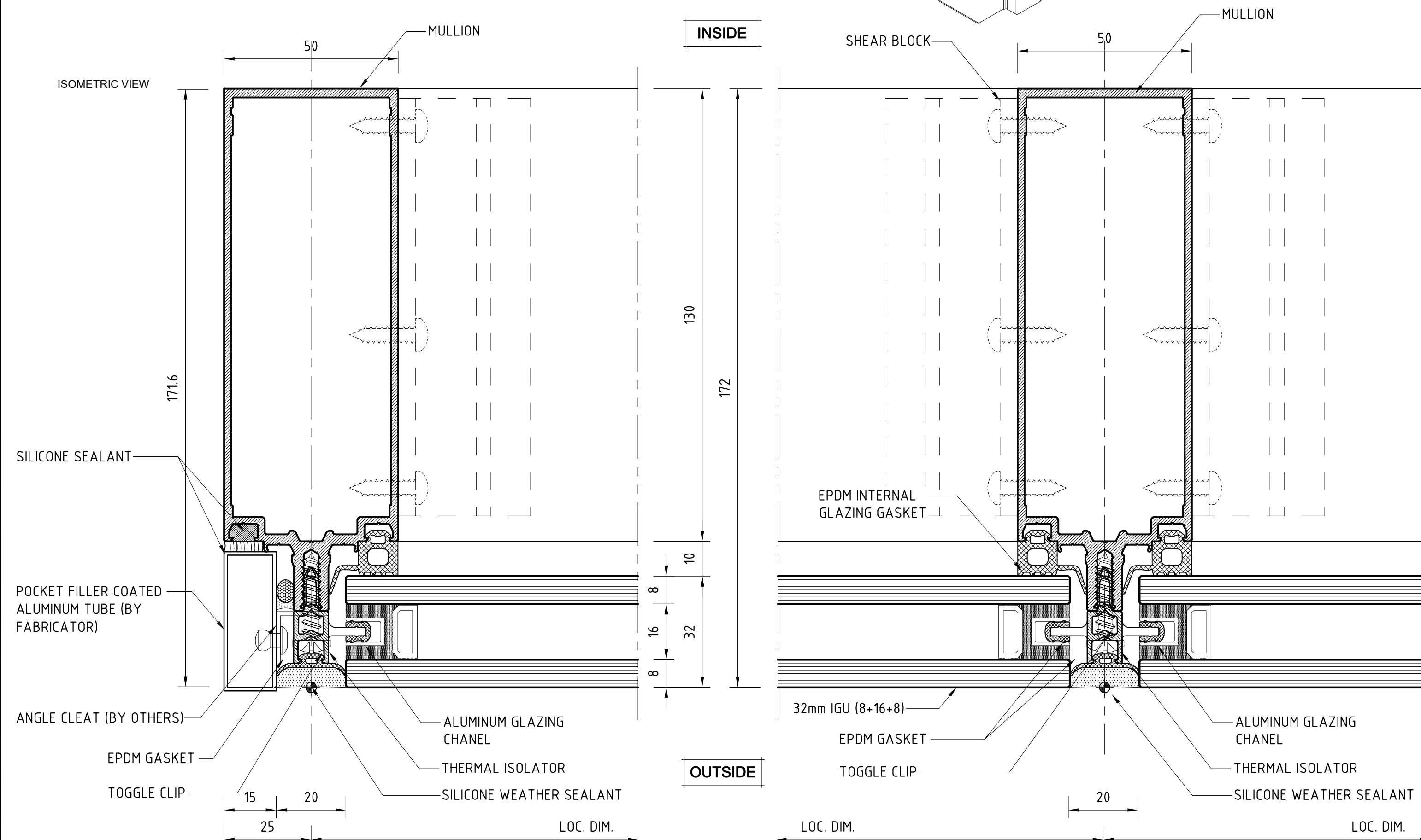
JAMB MULLION DETAIL
